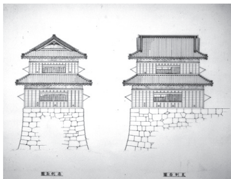
■上田城櫓移転設計図(昭和17年)
