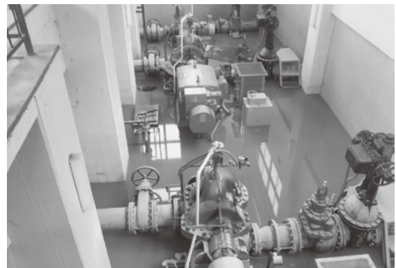
水没した川西揚水機場（農業用水の送水用ポンプ）
